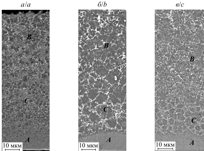
Рис. 1. Микроструктура поперечного сечения фольги исследуемых сплавов: a – сплав № 4; б – сплав № 3; в – сплав № 2
