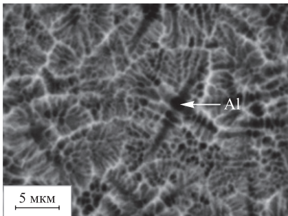
Рис. 2. Микроструктура и карта распределения кремния в слоях фольги сплава № 2: а, б – микроструктура слоя А при различном увеличении; в – микроструктура слоя В; г – распределение кремния в слое В
