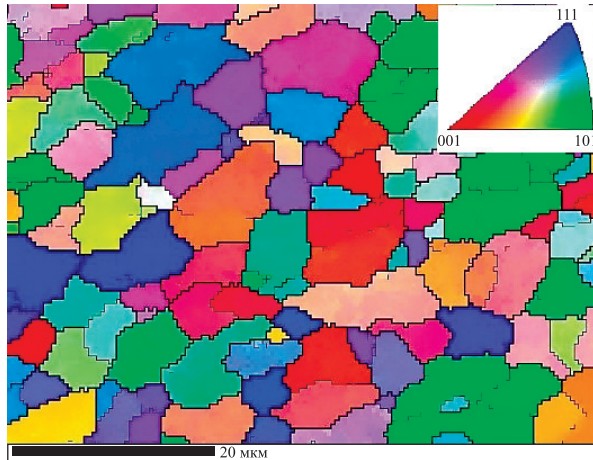
Рис. 3. Зеренная структура фольги сплава № 1:
