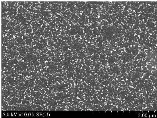
Рис. 3. РЭМ-изображение поверхности поликремния в структуре Al/poly-Si/SiO 2 /Si с удаленной пленкой алюминия после быстрой термообработки (450 °С, 7 с):
