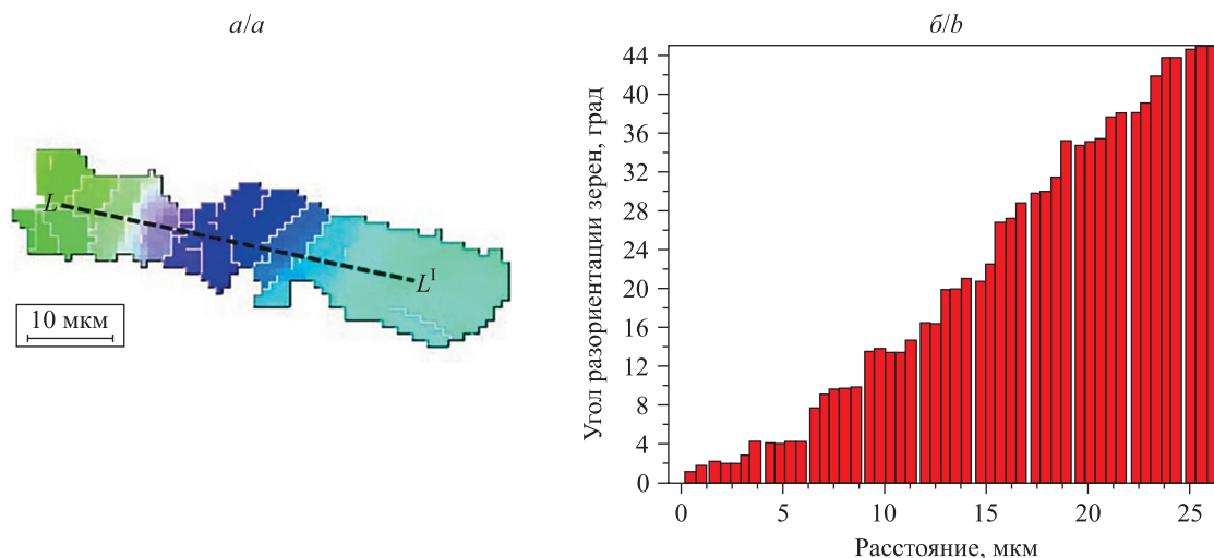
Рис. 6. Выбранное зерно фазы алюминия ( a ) и разориентация углов кристаллической решетки вдоль линии сканирования поверхности L-L' ( b )
