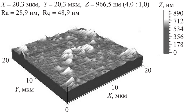
Рис. 4. АСМ-снимок наночастиц никеля Fig. 4. AFM image of nickel nanoparticles
