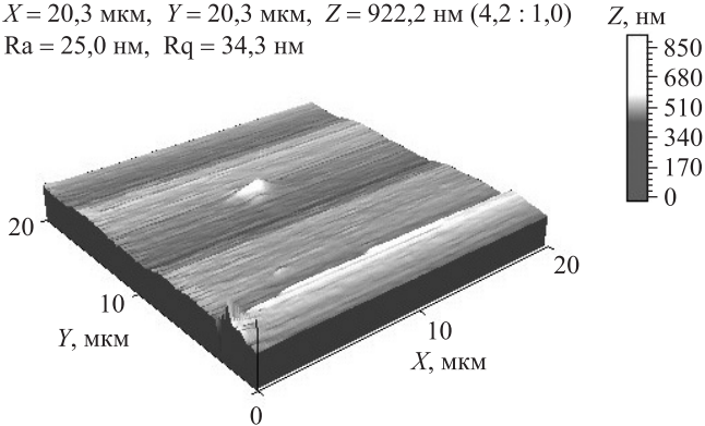
Рис. 5. АСМ-снимок наночастиц цинка
