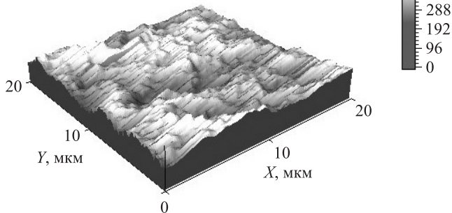
Рис. 6. АСМ-снимок наночастиц меди Fig. 6. AFM image of copper nanoparticles
