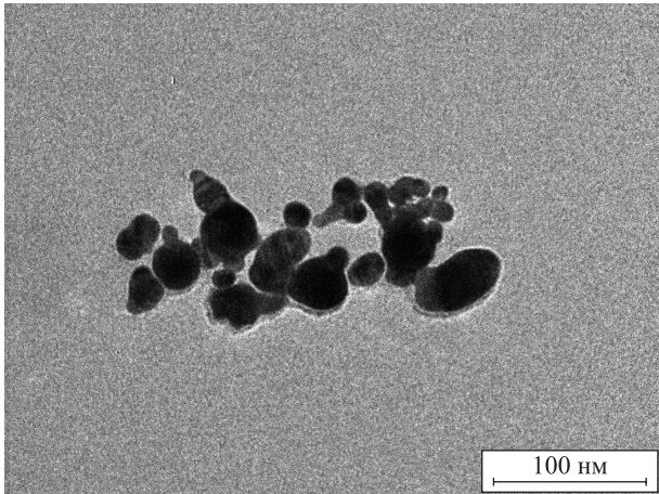
Рис. 10. ПЭМ-снимок наночастиц меди Fig. 10. TEM image of copper nanoparticles
