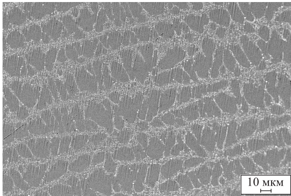
Рис. 2. Микроструктура светлых полос при масштабе 10 мкм (а) и масштабе 2 мкм (б)
