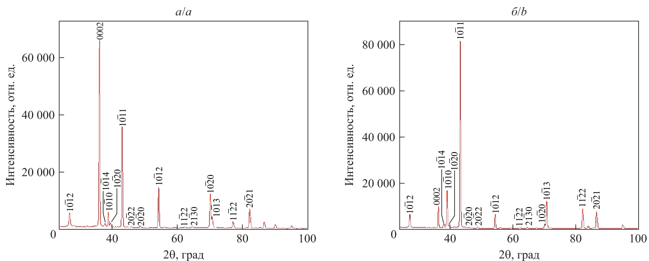
Рис. 7. Дифрактограммы быстрозатвердевшей фольги сплава Zn – 2 мас. % Bi для слоев, прилегающих к поверхности A (a) и поверхности B (б)
