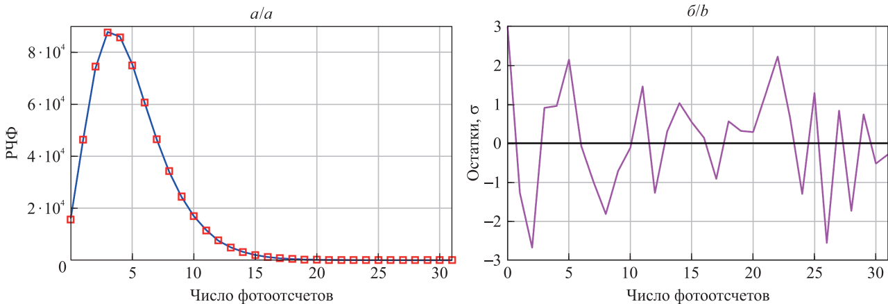
Рис. 4. Результаты анализа измеренных данных с использованием метода РЧН: a – экспериментальное (квадраты) и теоретическое (сплошная линия) РЧФ; b – график взвешенных остатков
