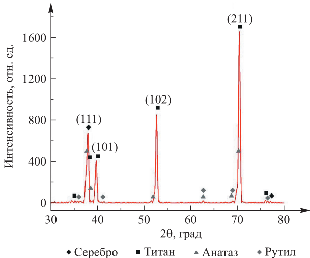
Рис. 2. Дифрактограмма гетероструктуры Ag/TiO 2 /Ti Fig. 2. Diffractogram of Ag/TiO 2 /Ti heterostructure
