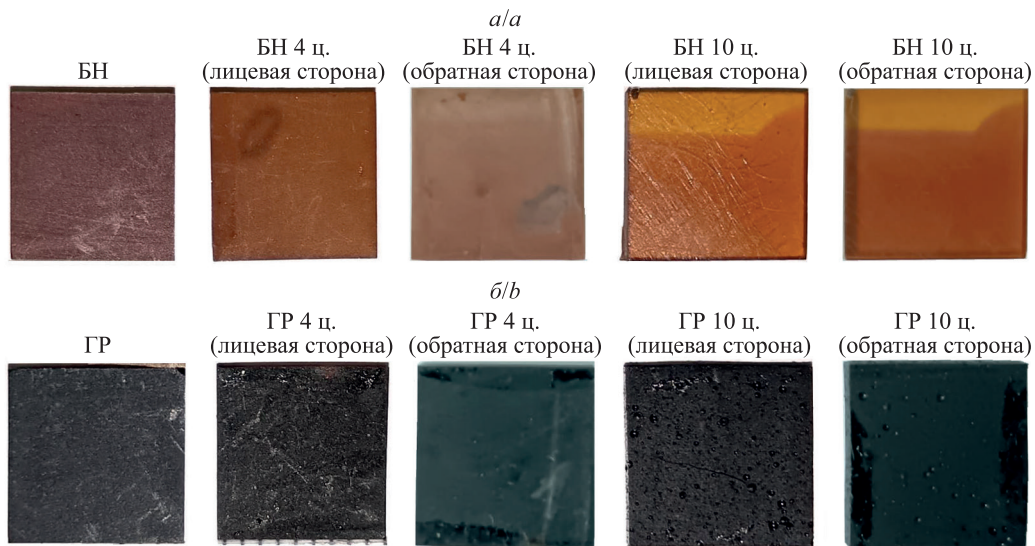
Рис. 2. Внешний вид лицевой (облученной) и обратной стороны образцов до и после 4 и 10 циклов ТЦ: a – образцы БН; б – образцы ГР
