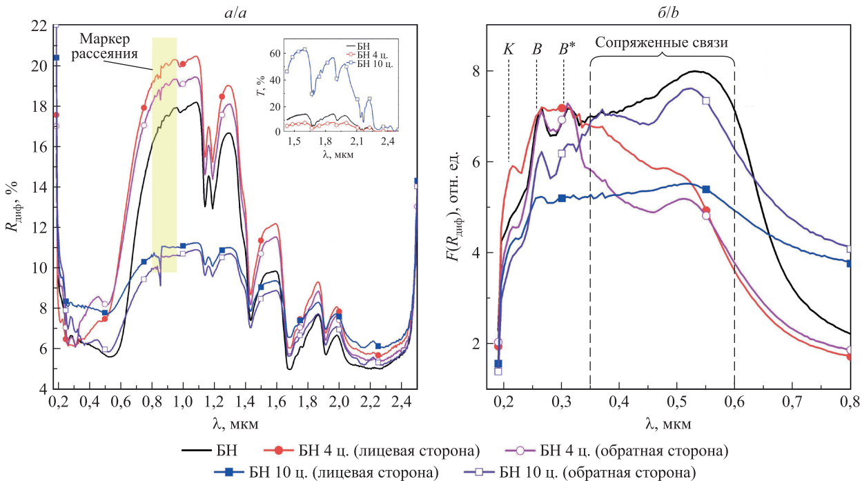
Рис. 4. Спектры диффузного отражения (а) и поглощения (б) для лицевой (облученной) и обратной стороны образцов БН до и после 4 и 10 циклов ТЦ Fig. 4. Diffuse reflection (a) and absorption (b) spectra for the front (irradiated) and back side of samples of unmodified polymer without filler before and after 4 and 10 cycles of TC
