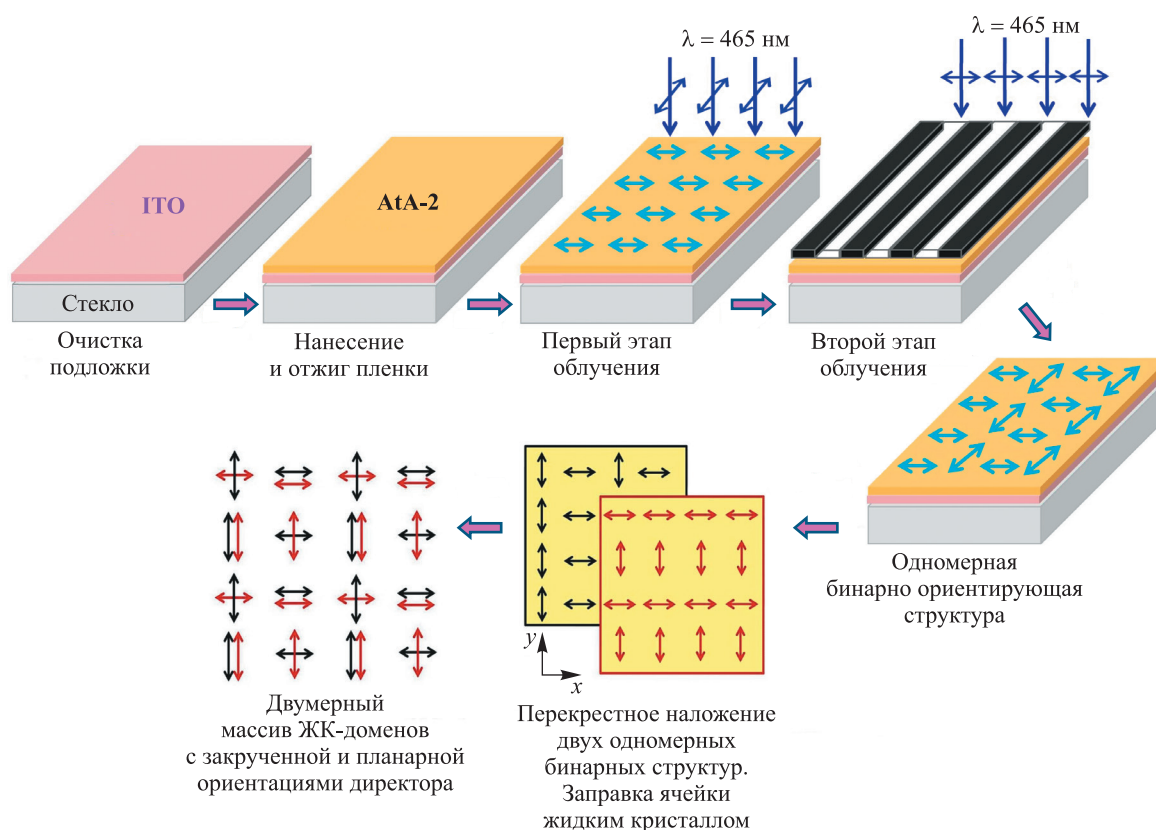
Рис. 2. Схема процесса формирования двумерного массива ЖК-доменов на основе технологии текстурированной фотоориентации
