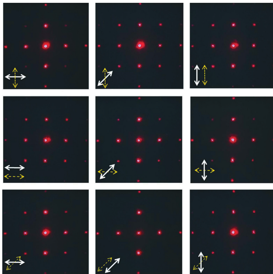
Рис. 4. Дифракционные картины, формируемые двумерной ЖК-решеткой в отсутствие напряжения. Пунктирной стрелкой показано направление поляризации падающего на решетку излучения, а сплошной стрелкой – направление оси ориентации анализатора
