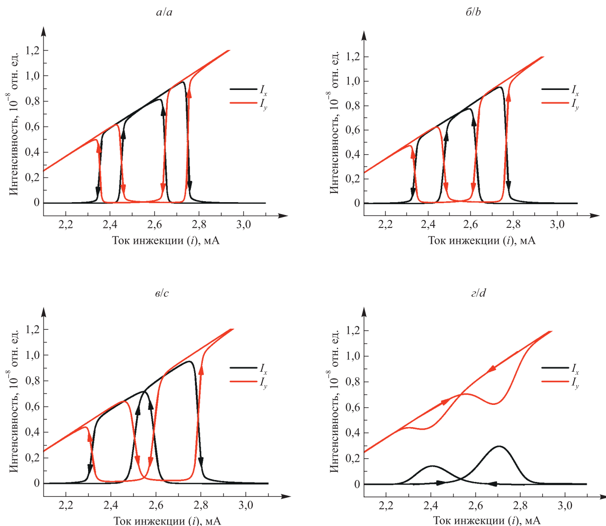
Рис. 7. Зависимость интенсивностей поляризационных мод I_x и I_y от величины тока инжекции при различных значениях коэффициента анизотропии: а – k_0 = 0,02 ; б – k_0 = 0,01 ; в – k_0 = 0,005 ; г – k_0 = 0,001 . Положение точек ПП: i_{ps1} = 2,4 мА, i_{ps2} = 2,7 мА. Время нарастания тока составляет 10^{-4} с
