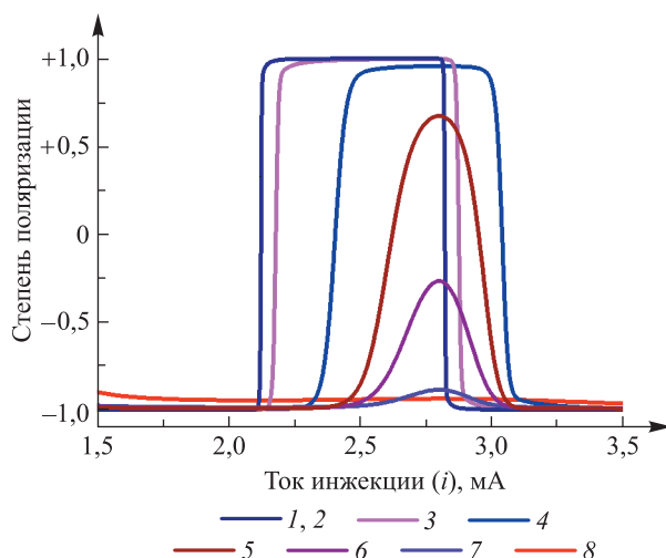
Рис. 2. Зависимость степени поляризации выходного излучения от величины тока инжекции при различных скоростях его нарастания.
