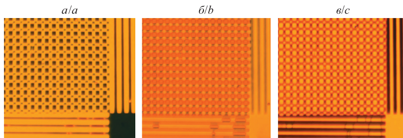
Рис. 3. Поляризационные микрофотографии фазовой дифракционной решетки на основе двумерного массива ЖК-доменов (период структуры 20 мкм): a – оси поляризатора и анализатора параллельны; б – оси поляризатора и анализатора ориентированы под углом 45^\circ ; в – оси поляризатора и анализатора скрещены
