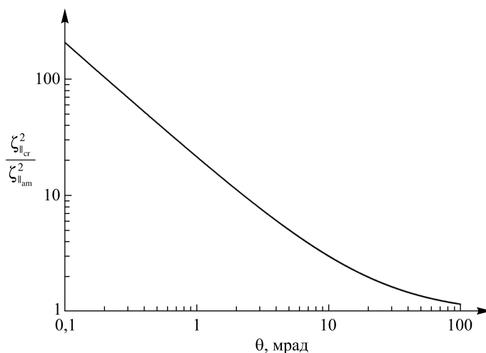
Рис. 2. Зависимость отношения квадратов продольной поляризации, приобретаемой тяжелыми барионами в кристалле и аморфном веществе, от угла, образуемого их импульсами с осью \langle 111 \rangle кристалла вольфрама
