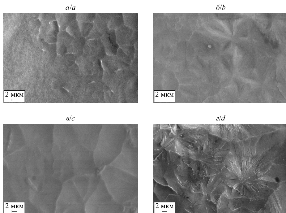
Рис. 4. РЭМ-изображения поверхности циркония
