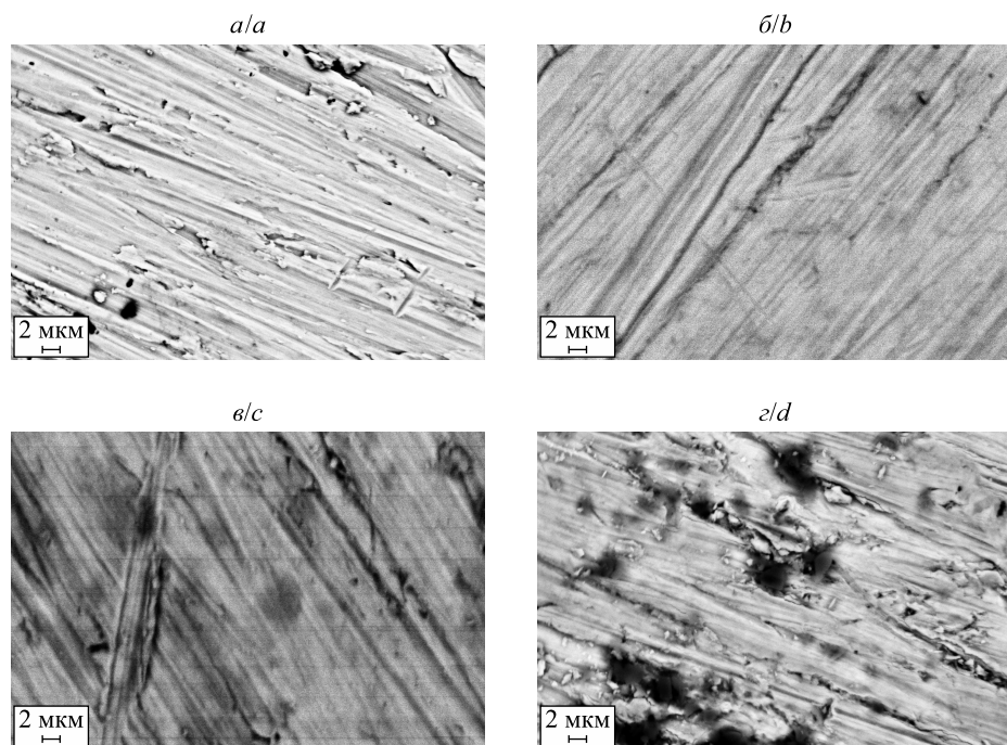
Рис. 3. РЭМ-изображения поверхности циркония после высокотемпературного отжига:
