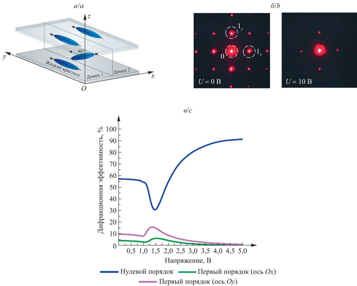
Рис. 5. Дифракционные свойства переключаемой двумерной ЖК-решетки с закрученной и планарной ориентациями директора жидкого кристалла:
