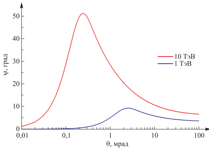
Рис. 3. Зависимость угла поворота вектора поляризации, приобретаемого нейтральным очарованным омега-барионом с энергиями 1 и 10 ТэВ в кристалле вольфрама толщиной 3 и 10 см, от угла, образуемого импульсом бариона с осью \langle 111 \rangle кристалла вольфрама
